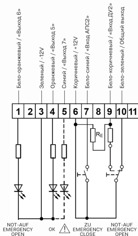
Кнопка HSE производства AUMULLER
