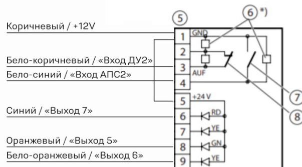
Кнопка RWA-Taster FT4/24 V DC производства GEZE
