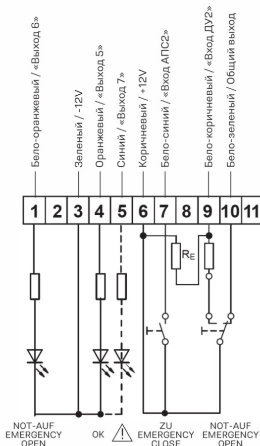
Кнопка HSE производства AUMULLER
