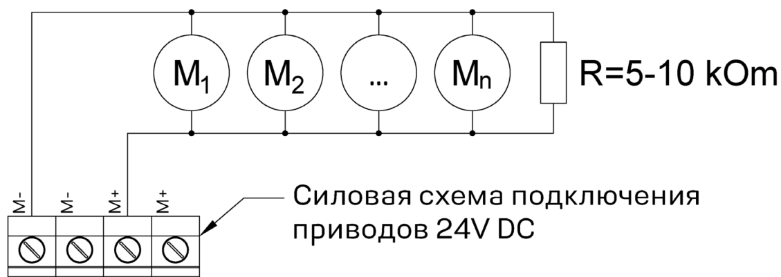
Рис. 4. Схема подключения приводов 24V DC
