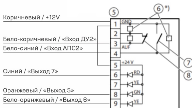
Кнопка RWA-Taster FT4/24 V DC производства GEZE
