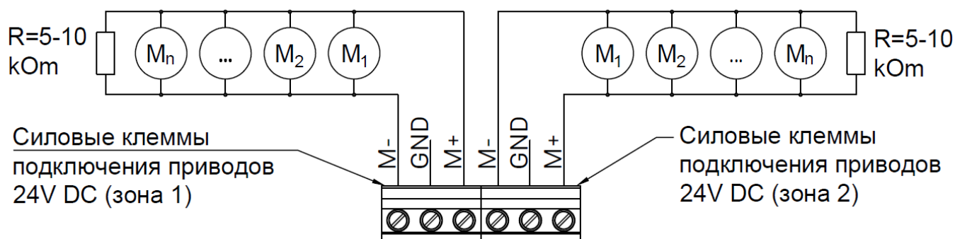
Рис. 4. Схема подключения приводов 24V DC
