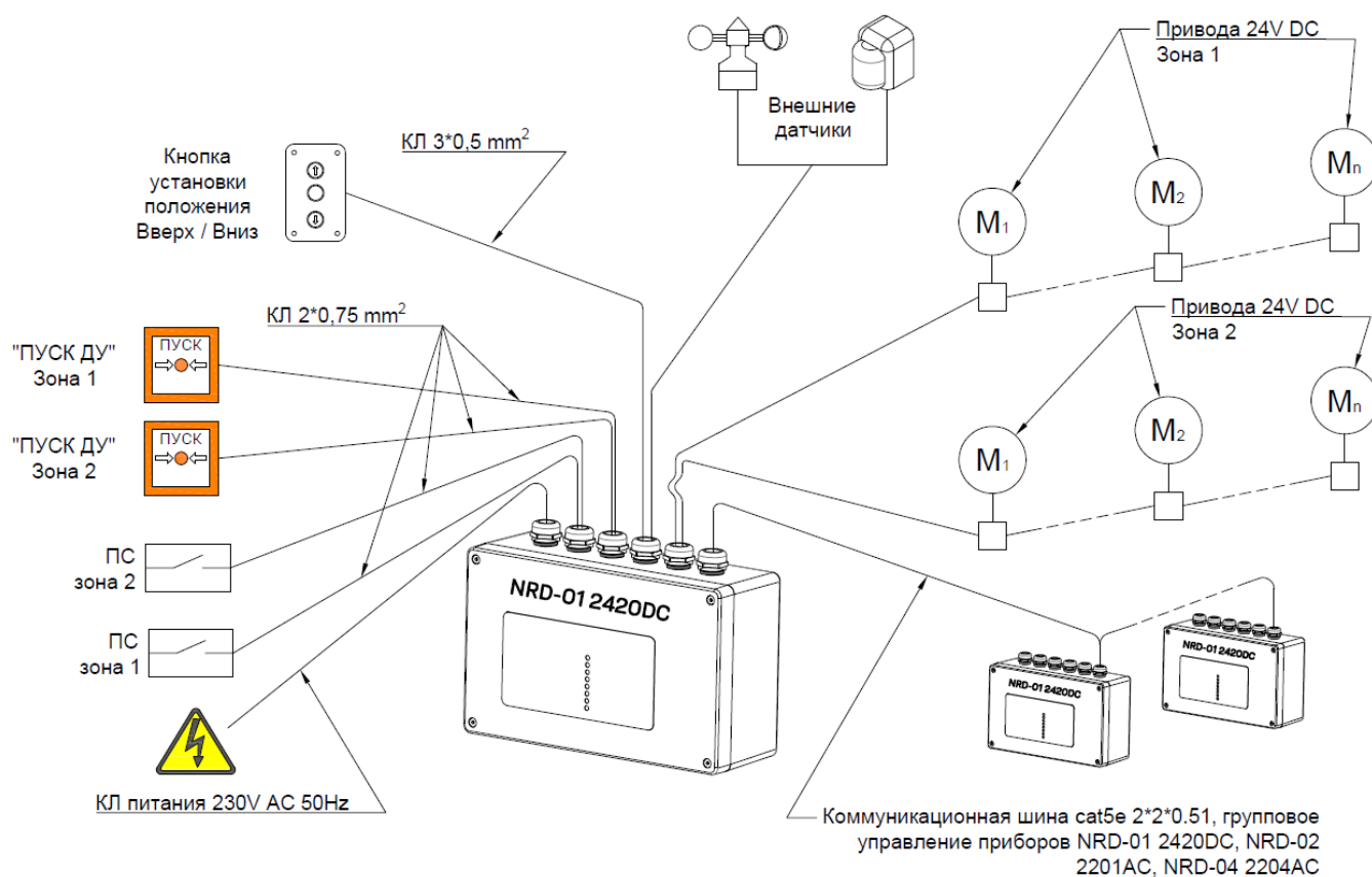
Рис. 3. Схема прокладки кабельных линий
