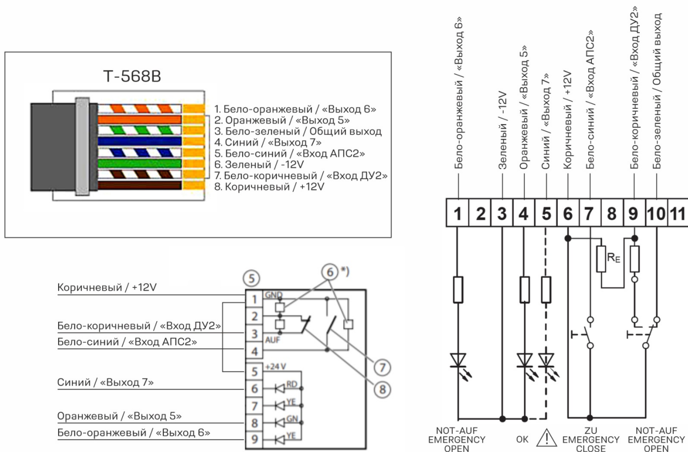
Кнопка RWA-Taster FT4/24 V DC производства GEZE
