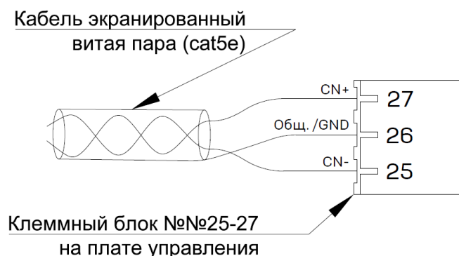
Рис. 8. Схема подключения коммуникационной шины (групповое управление).
