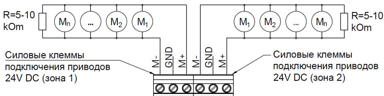
Рис. 4. Схема подключения приводов 24V DC
